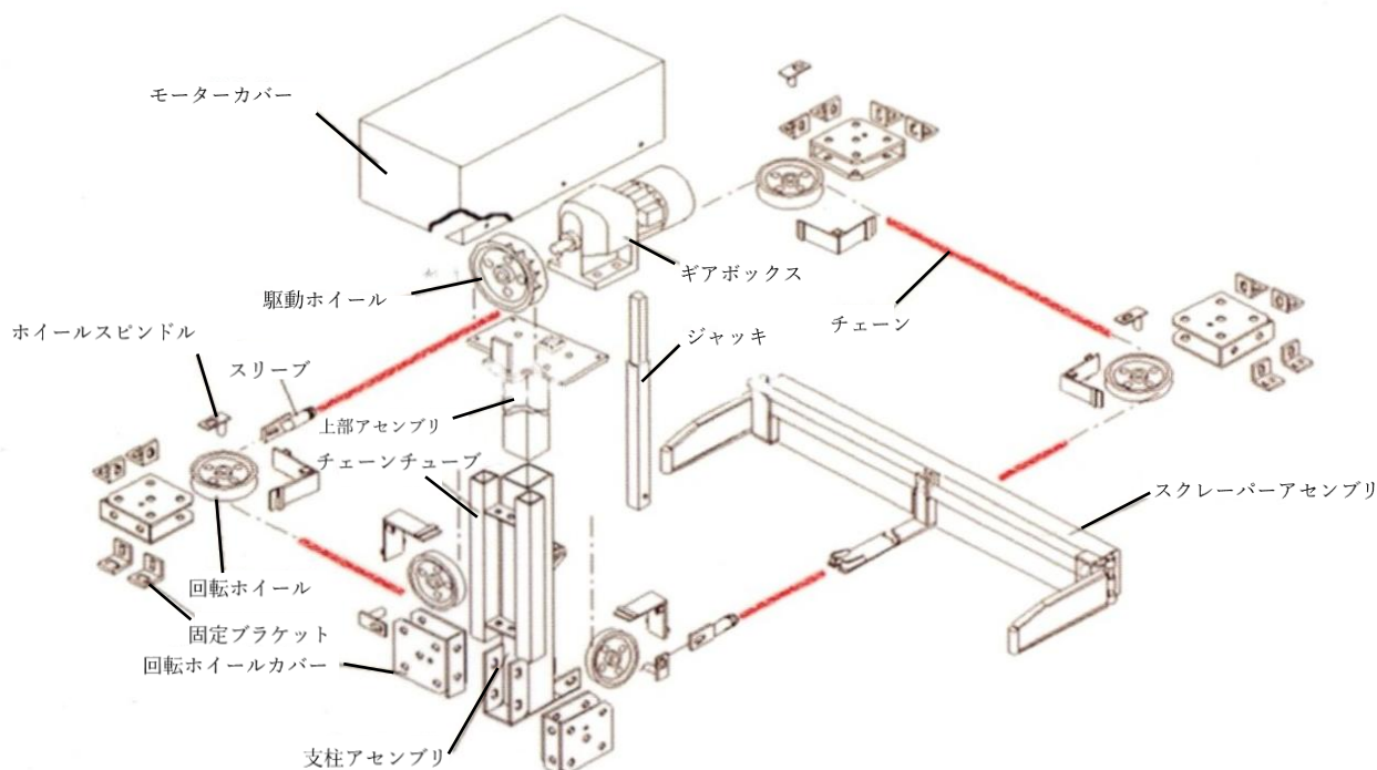
1・牛舎自動糞尿スクレーパー配置図
