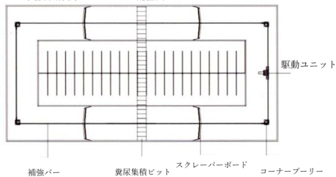
2・牛舎自動糞尿スクレーパー配置図
