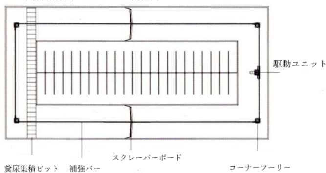
1・牛舎自動糞尿スクレーパー配置図
